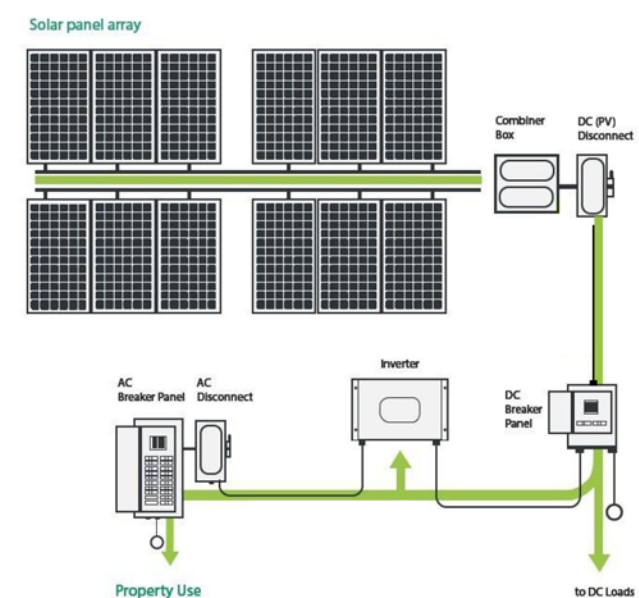
HỆ THỐNG NĂNG LƯỢNG MẶT TRỜI ĐỘC LẬP / OFF-GRID SOLAR SYSTEM
