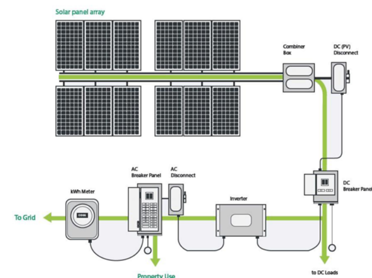
HỆ THỐNG NĂNG LƯỢNG MẶT TRỜI HÒA LƯỚI / ON-GRID SOLAR SYSTEM
